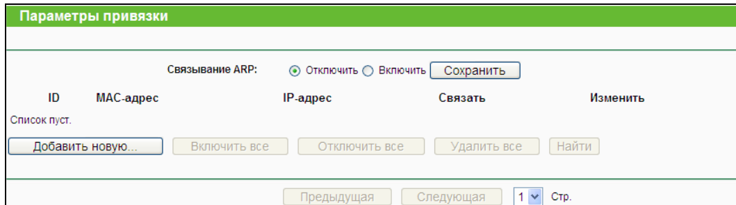
Рис. 4-83 Параметры привязки
