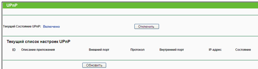
Рис. 4-50 UPnP
