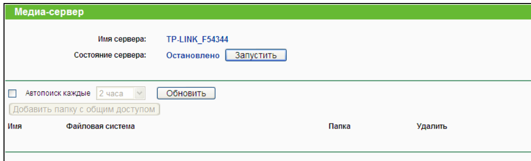
Рис. 4-38 Медиа-сервер
