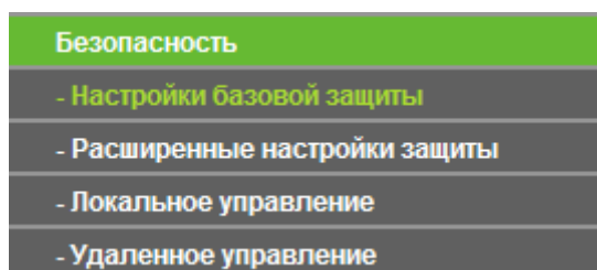
Рис. 4-51 Меню Безопасность
