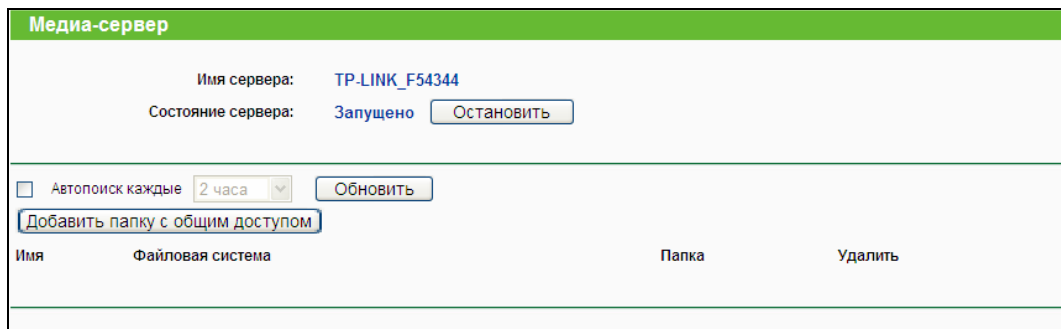
Рис. 4-39 Медиа-сервер
