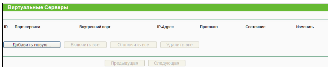
Рис. 4-45 Виртуальные серверы
