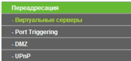
Рис. 4-44 Меню Переадресация
