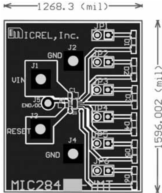
Top Layer
