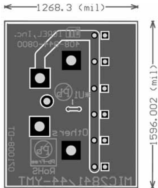
Bottom Layer
