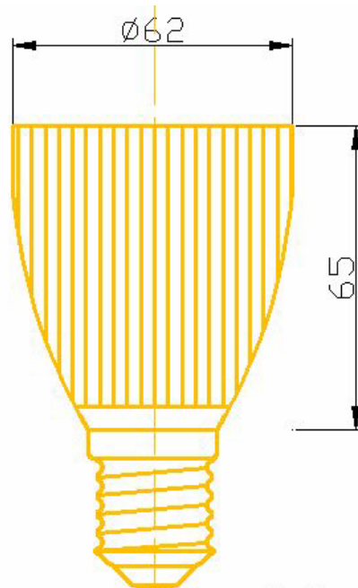
Unit:mm RP-SL-E03-5WXXE27
