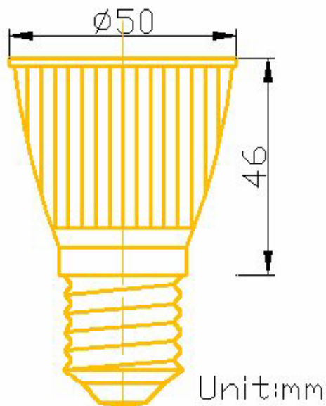
RP-SL-E01-3WXXE27
