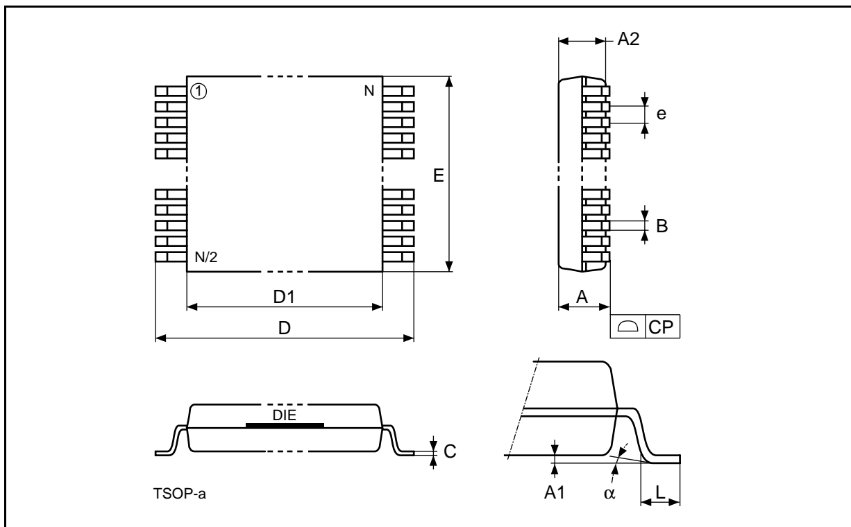
TSOP56
