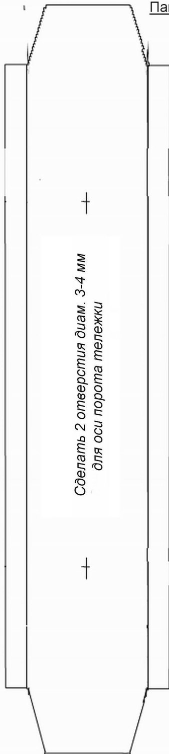
Рама (1 дет.)
